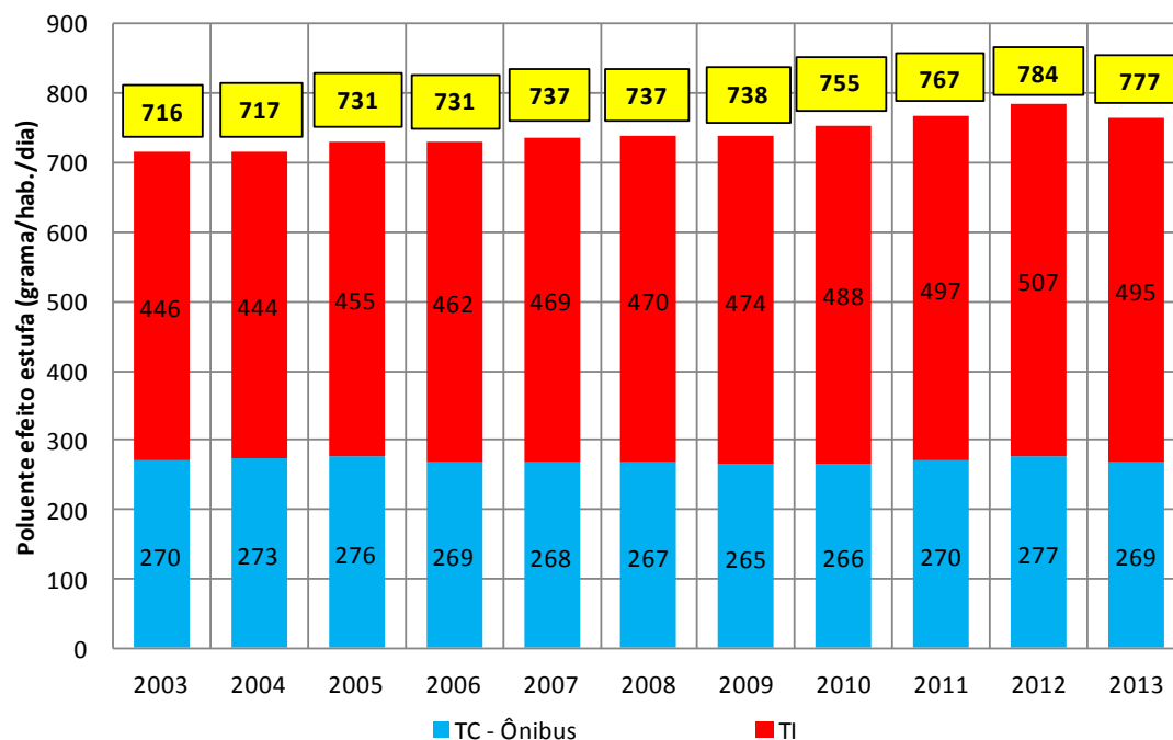
Gráfico 30 – Emissões de poluente estufa por habitante por dia, por modo agregado (grama por habitante/dia)
