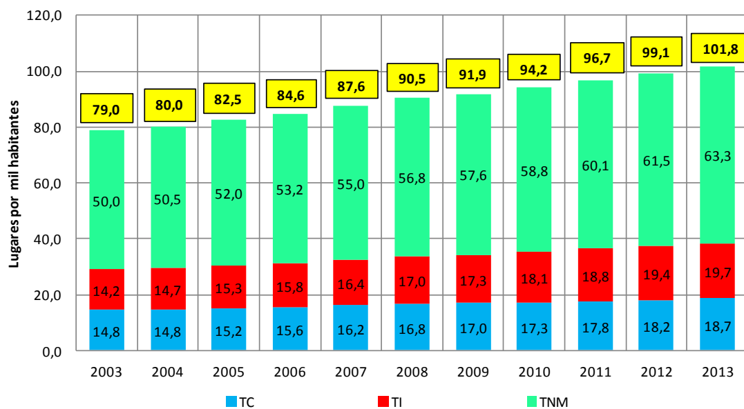
Gráfico 14 – Total de deslocamentos, por modo agregado 8
