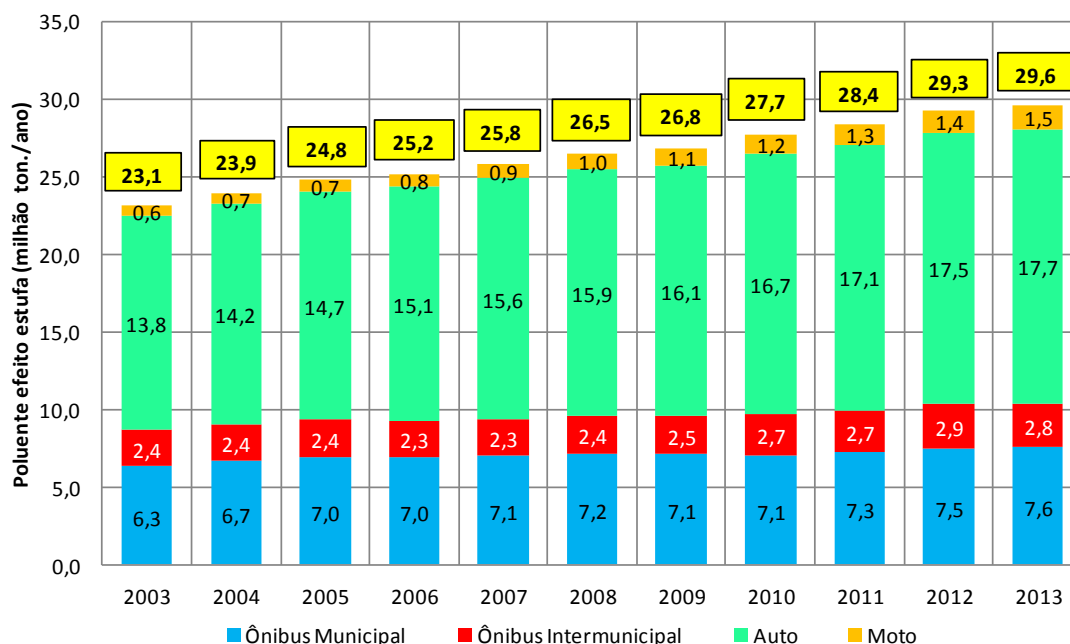
Gráfico 29 – Emissões de poluente estufa por modo (milhão ton./ano)
