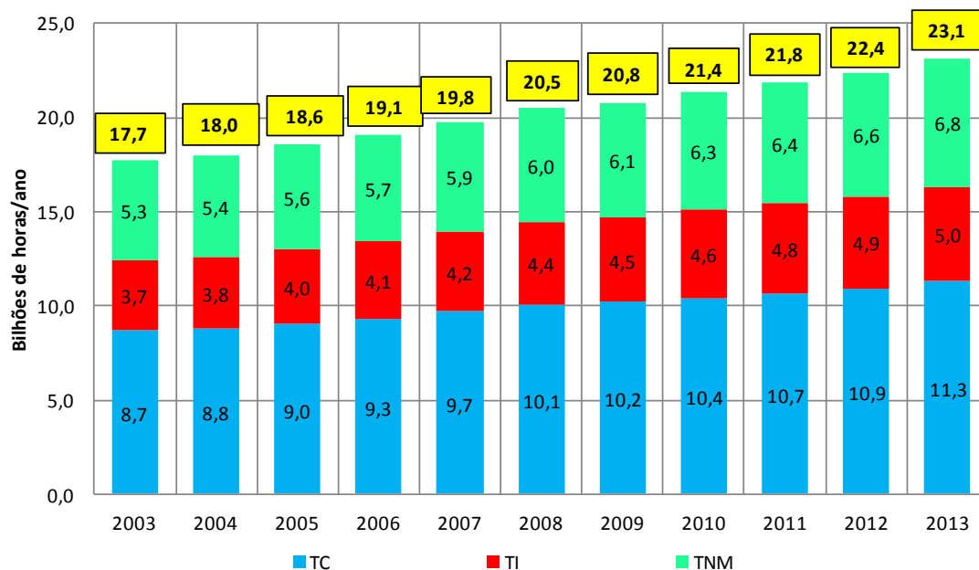
Gráfico 20 – Consumo de tempo na mobilidade, por modo agregado (bilhões de horas/ano)
