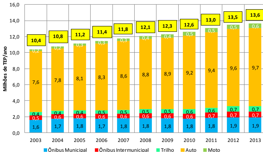
Gráfico 22 – Evolução da quantidade de energia consumida na mobilidade urbana por modo (milhões de TEP/ano)
