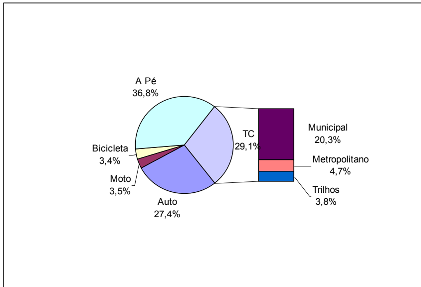
Gráfico 5 – Divisão modal – 2011
